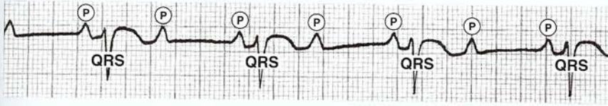
2:1 Mobitz AV block
